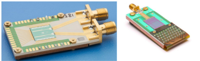
Obr. 10: Realizácia Josephsonovho sériového poľa JAWS (vľavo) a PJVS (vpravo) [5].
