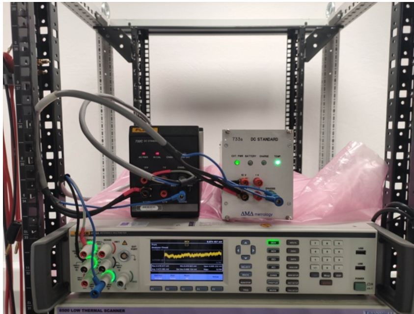
Obr. 90: Porovnanie etalónu voči Fluke 732C-S.
