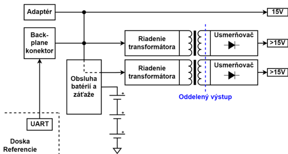
Obr. 17: Bloková schéma napájacej časti etalónu.
