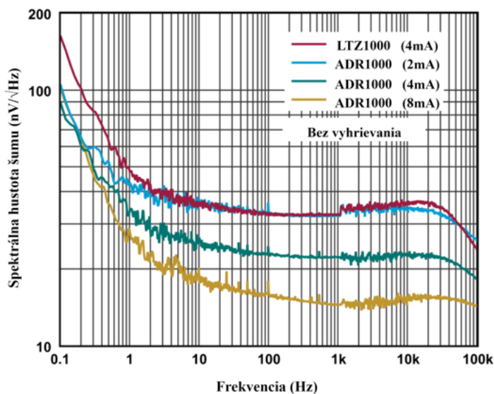
Obr. 21: Porovnanie šumu ADR1000 a LTZ1000 pri rôznych úrovniach záťaže bez zapnutého vyhrievania [8].
