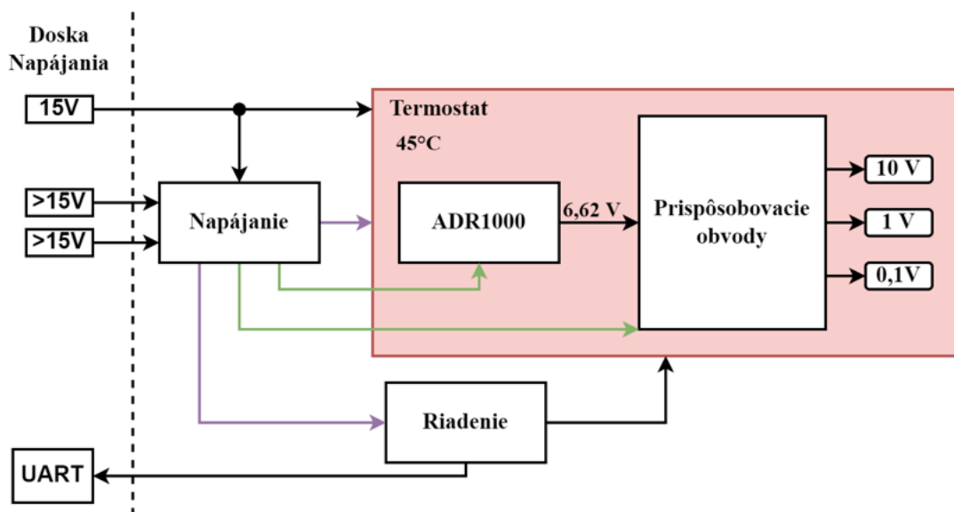
Obr. 18: Bloková schéma referenčnej časti etalónu.
