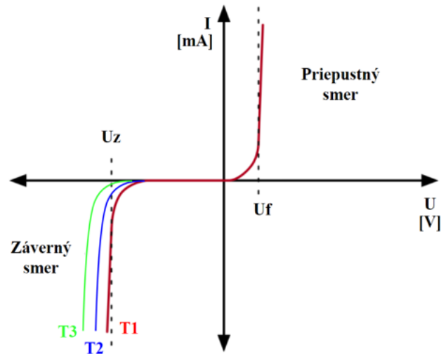
Obr. 3: Volt-Ampérová charakteristika Zenerovej diódy so znázornenou hranicou Zenerovho prierazu U_z v závernom smere. Na obrázku tiež môžeme vidieť že pri zmene teploty T (znázornené ako T_1 , T_2 a T_3 ) dochádza k posunutiu hranice Zenerovho prierazu.
