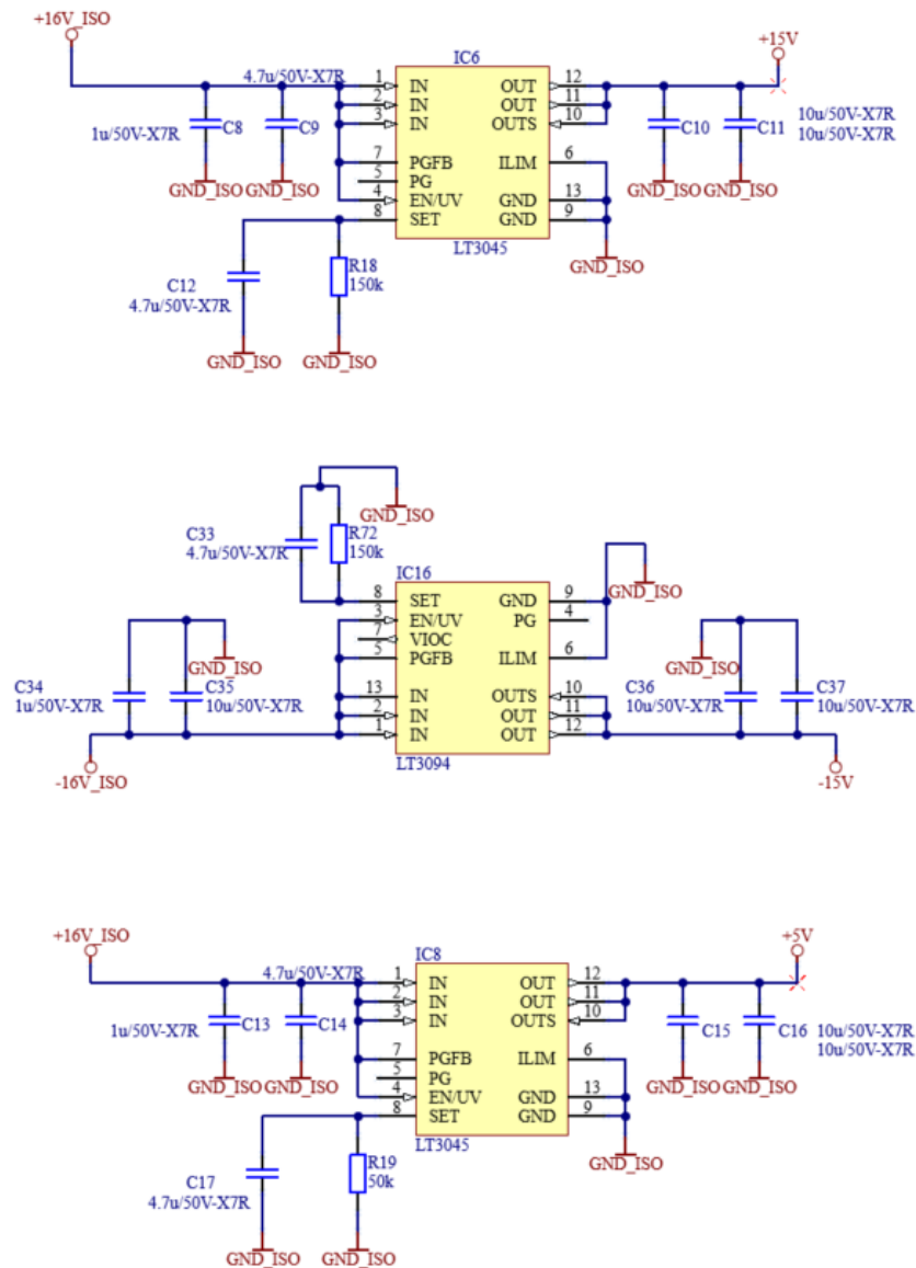
Obr. 47: Schéma lineárnych stabilizátorov pre galvanicky oddelené napájacie vetvy.
