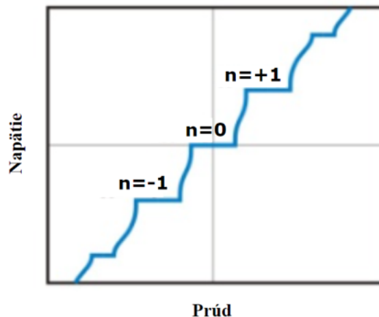
Obr. 8: Konštantné napätové kroky volt-ampérovej charakteristiky Josephsonových prechodov [4].
