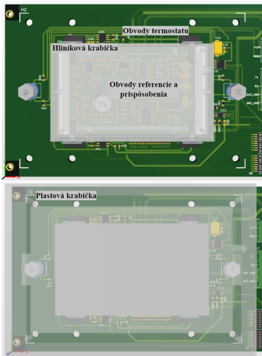
Obr. 30: Architektúra termostatu.
