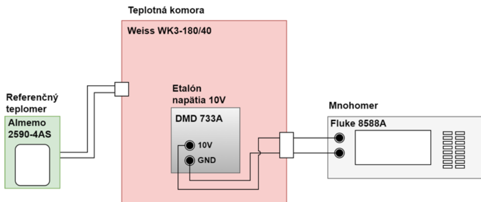
Obr. 85: Principiálna schéma pre meranie teplotnej stability.
